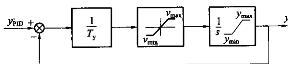
c) 电液随动系统模型之三
