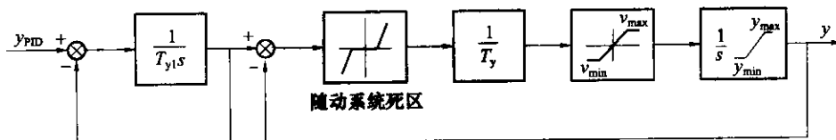
d) 电液随动系统模型之四
