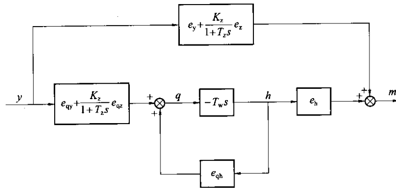
a) 转桨式水轮机模型之一
