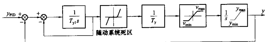
a) 电液随动系统模型之一
