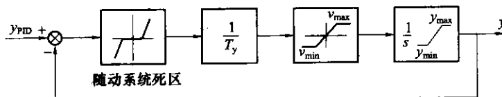
b) 电液随动系统模型之二
