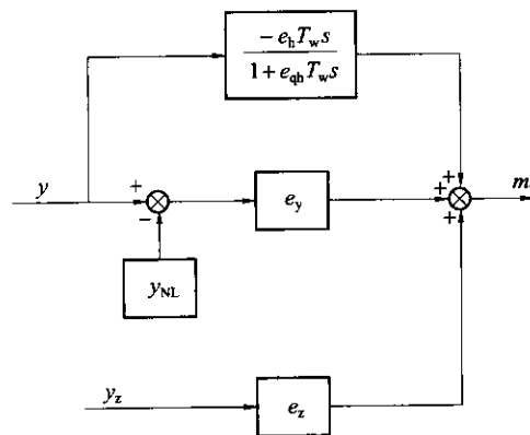
b) 转桨式水轮机模型之二
