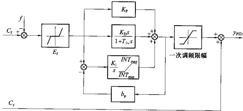
b) 调节器模型之二
