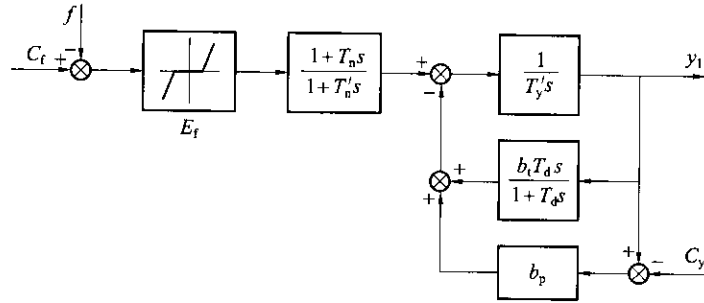
a) 调节器模型之一
