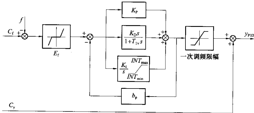
c) 调节器模型之三
